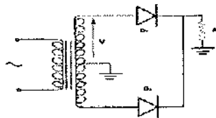
Gambar 2.12 Rangkaian penyearah gelombang penuh 2 diode
