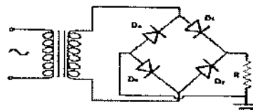
Gambar 2.10 Rangkain penyearah gelombang penuh ( Full Wave Rectifier )
