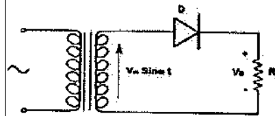
Gambar 2.8 Penyearah setengah gelombang ( Half Wave Rectifier )
