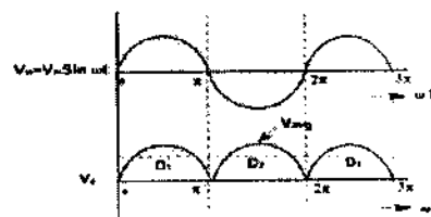
Gambar 2.13 Sinyal output penyearah gelombang penuh
